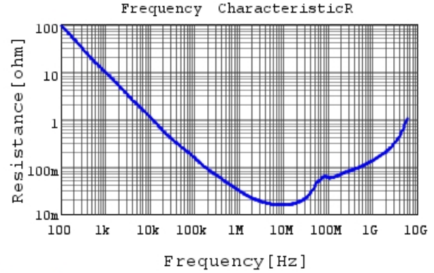
GRM155B31H104KE14 R DCOV, 20degC
