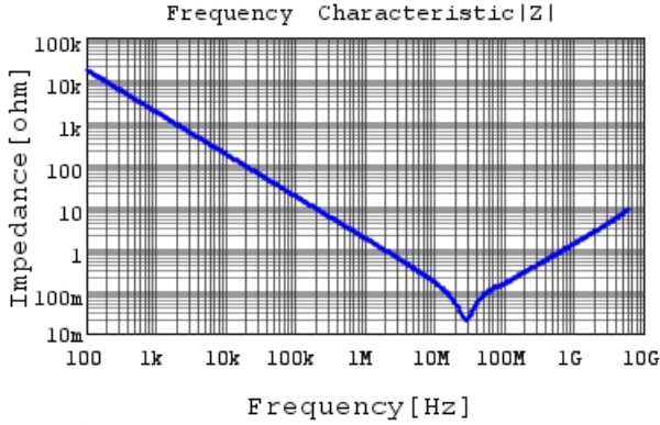
GRM155B31H104KE14 |Z| DCOV, 20degC
