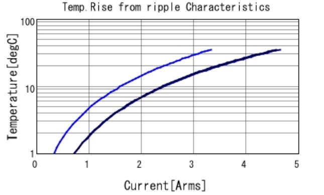
GRM319R61H475KA12 Temp. rise — 100kHz — 500
