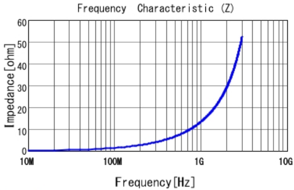
LQG15HH2N2C02 |Z|
