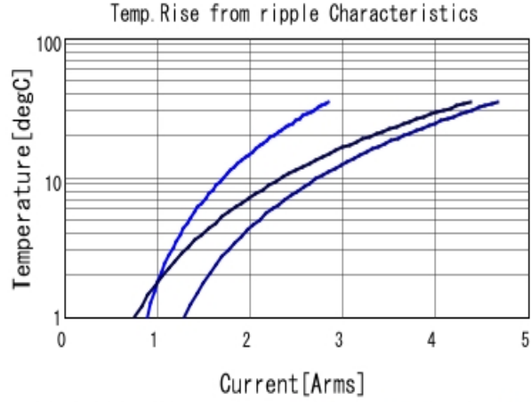
■ GRT31CR71H225KE13 Temp. rise ■ 100kHz ■ 500kHz ■ 1MHz
