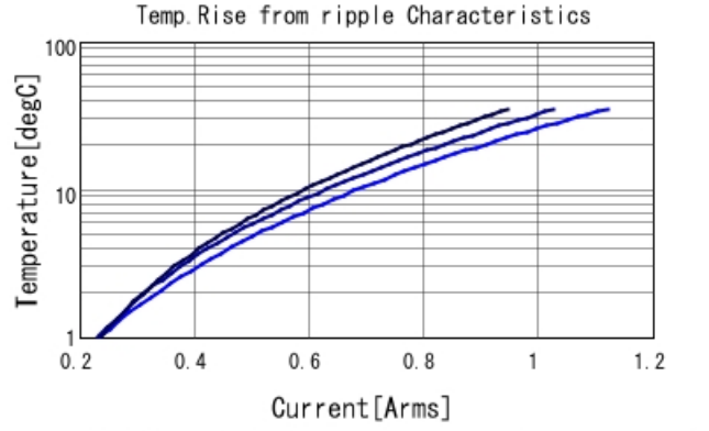
GRM1555C1H130JA01 Temp. rise — 500MHz — 700I
