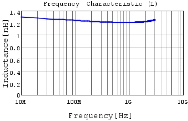
LQG15HN1N2S02 L
