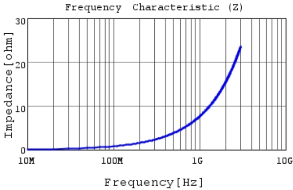
LQG15HN1N2S02 |Z|
