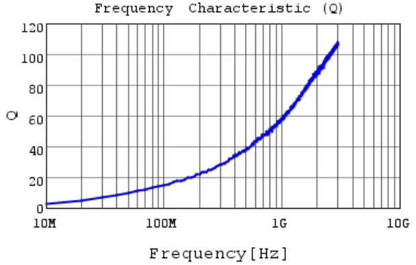
LQG15HN1N2S02 Q
