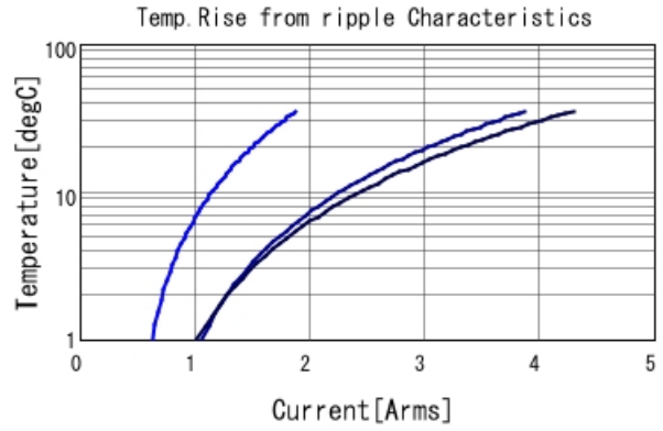
GRM21BR71C105KA01 Temp. rise — 100kHz — 500
