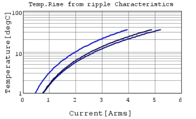
GRM31CC72A475ME11 Temp.rise — 100kHz —
