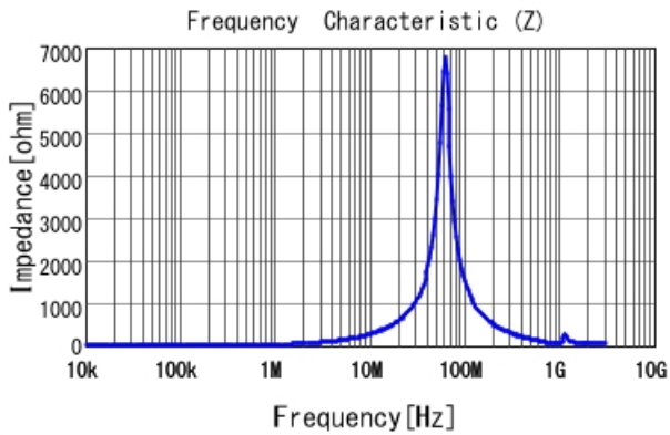
#A921CY-4R7M=P3 |Z|
