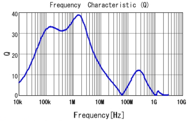
#A921CY-4R7M=P3 Q
