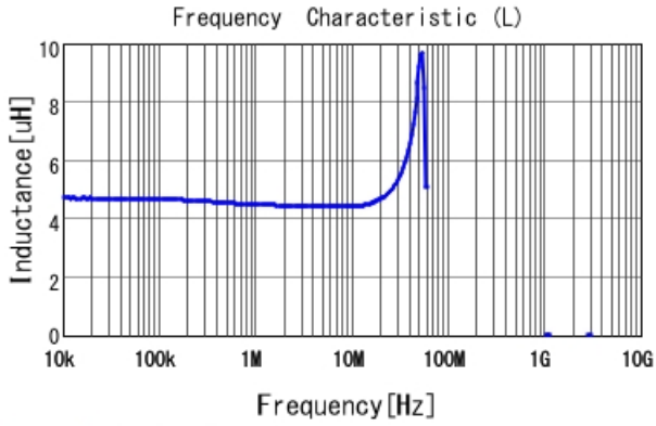
#A921CY-4R7M=P3 L
