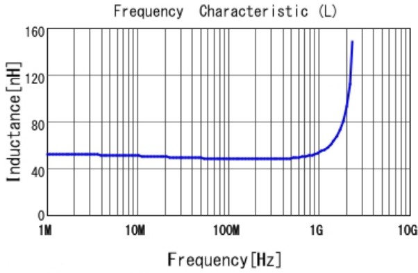
LQW18AN48NG8Z L
