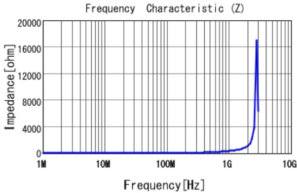
LQW18AN48NG8Z |Z|
