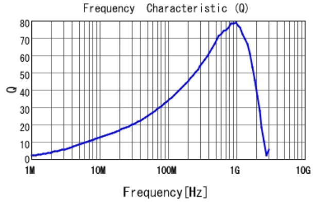
LQW18AN48NG8Z Q
