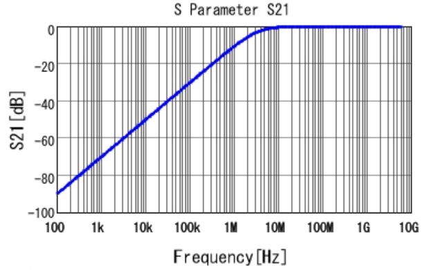
■ GRM033R71H471KA12 S21 DCOV, 25degC
