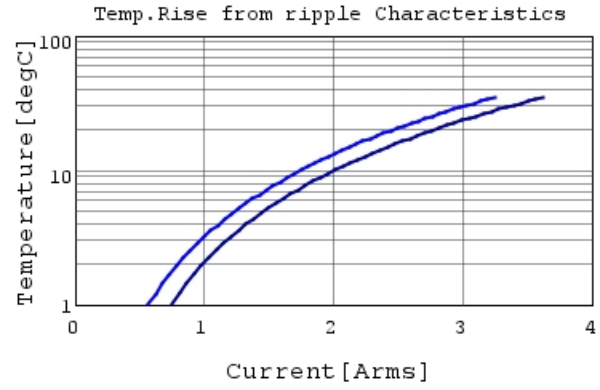
GRM155C70J225ME11 Temp.rise — 500kHz
