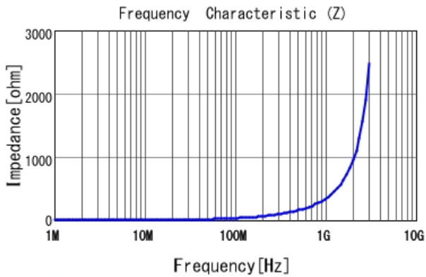
LQW15AN51NJ8Z |Z|
