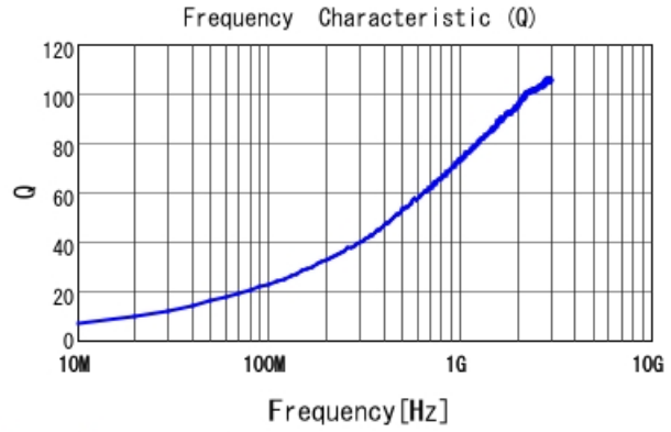
LQW15AN5N2D10 Q
