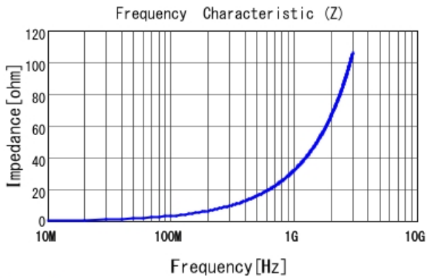
LQW15AN5N2D10 |Z|
