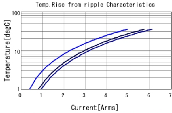
GRT31CC80J476KE13 Temp. rise ■ 60kHz ■ 300kHz ■ 600kHz
