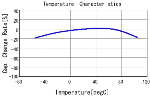
■ GRT31CC80J476KE13 C-Temp. capchange, DCO. 0V, ACO. 5Vrm
