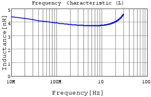
LQG15HZ3N9S02 L
