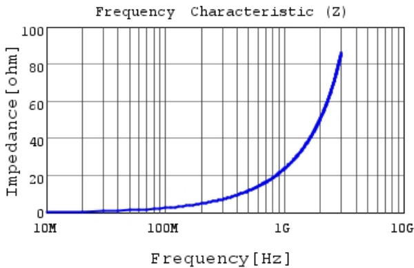
LQG15HZ3N9S02 |Z|
