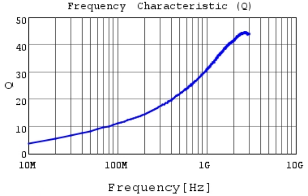
LQG15HZ3N9S02 Q
