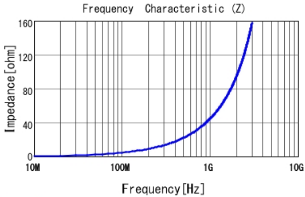
LQW15AN7N2G00 |Z|
