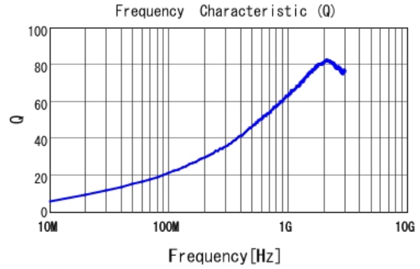
LQW15AN7N2G00 Q
