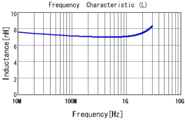
LQW15AN7N2G00 L
