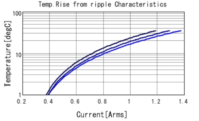
GJM1555C1H220GB01 Temp. rise — 500MHz — 700I
