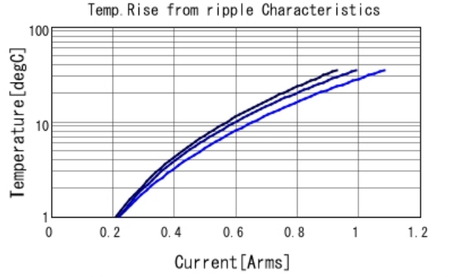
GRM1555C1H160JA01 Temp. rise — 500MHz — 700I
