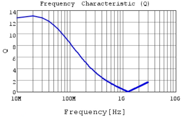
LQW18CNR39J00 Q
