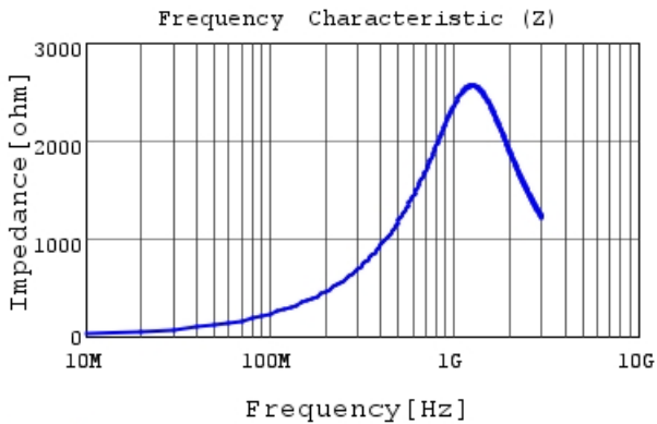
LQW18CNR39J00 |Z|
