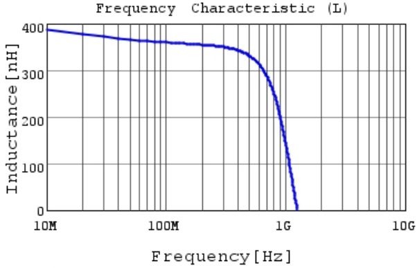
LQW18CNR39J00 L
