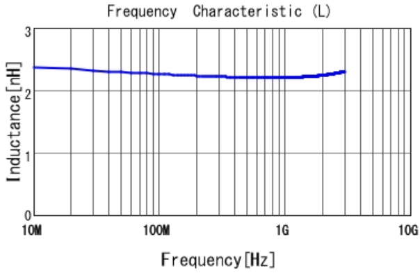
LQW15AN2N4B0Z L
