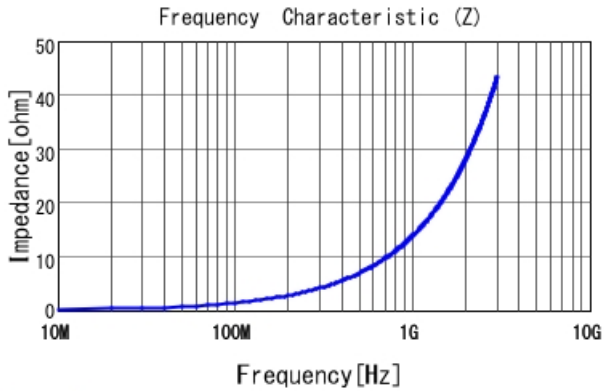
LQW15AN2N4B0Z |Z|
