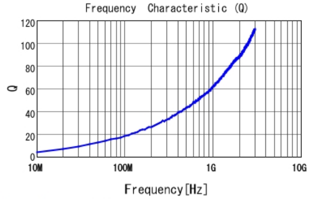
LQW15AN2N4B0Z Q
