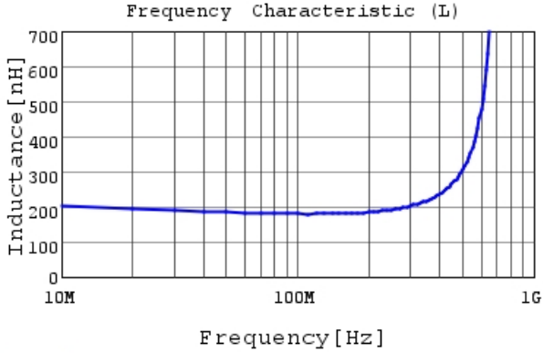
LQG15HSR18H02 L
