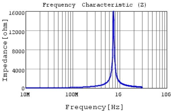
LQG15HSR18H02 |Z|
