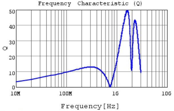
LQG15HSR18H02 Q
