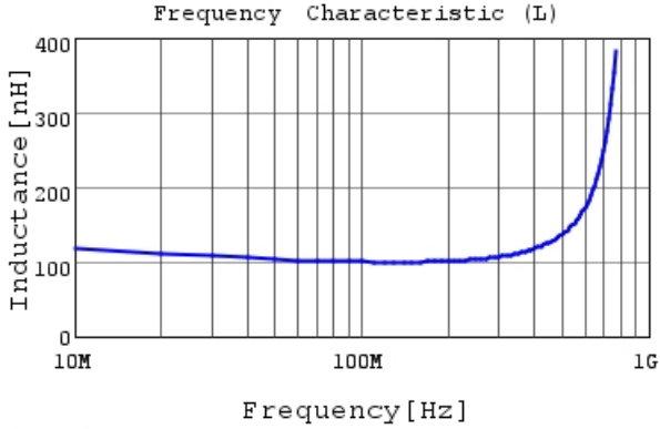
LQG15HNR10J02 L
