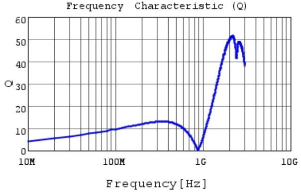
LQG15HNR10J02 Q
