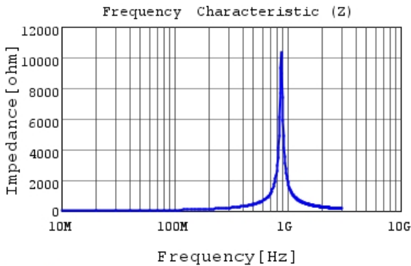
LQG15HNR10J02 |Z|
