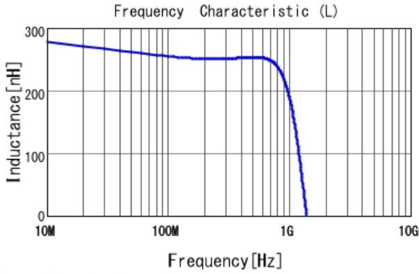
LQW15CAR27K00 L
