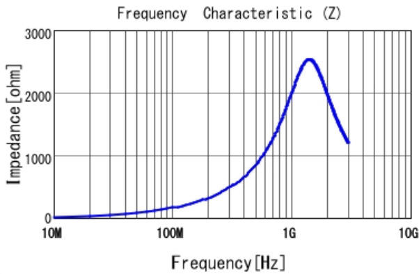
LQW15CAR27K00 |Z|
