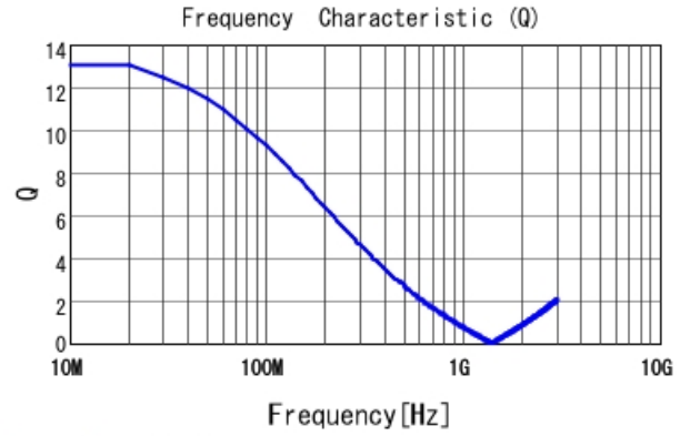
LQW15CAR27K00 Q
