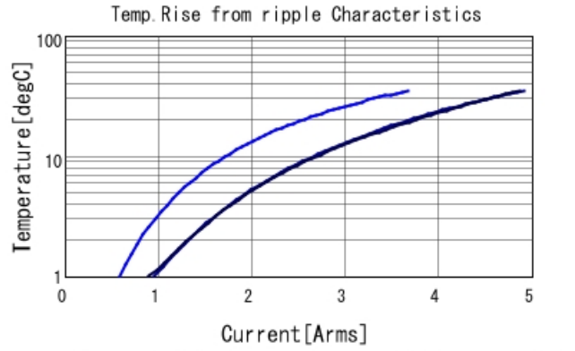
GRM319B30J106KE18 Temp. rise — 100kHz — 500
