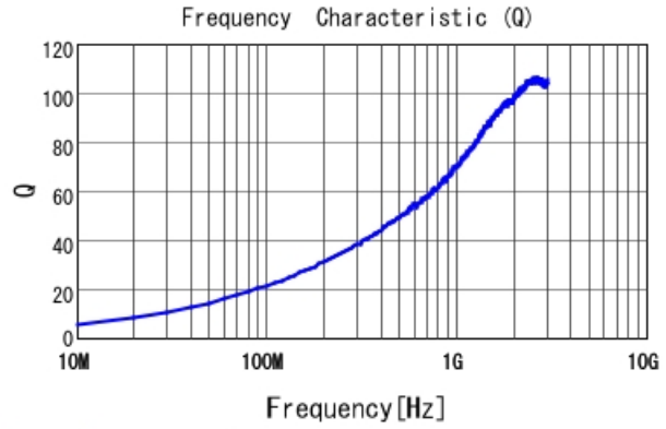
LQW15AN5N6C1Z Q
