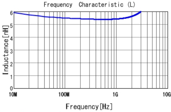
LQW15AN5N6C1Z L
