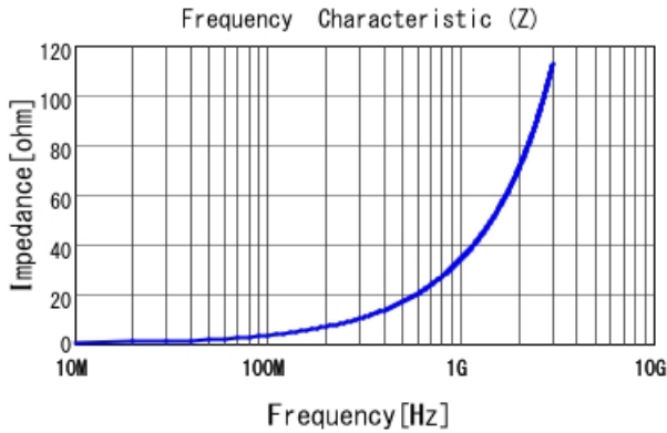
LQW15AN5N6C1Z |Z|
