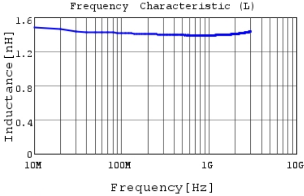
LQW15AN1N5C00 L
