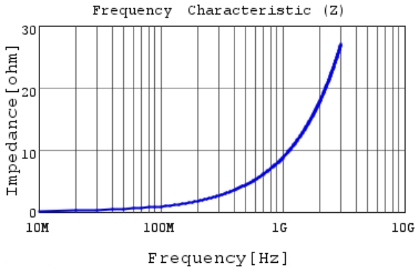
LQW15AN1N5C00 |Z|
