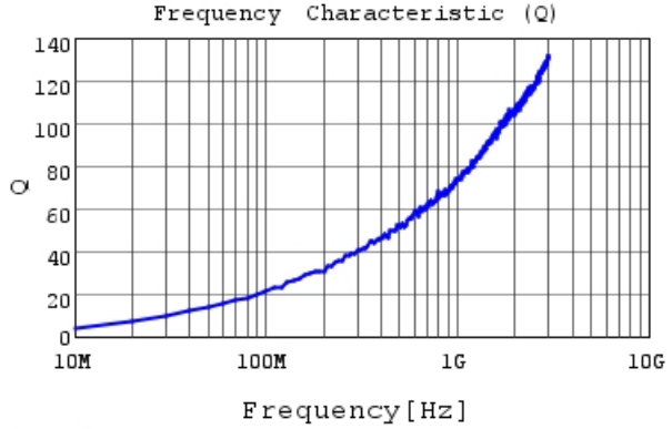
LQW15AN1N5C00 Q
