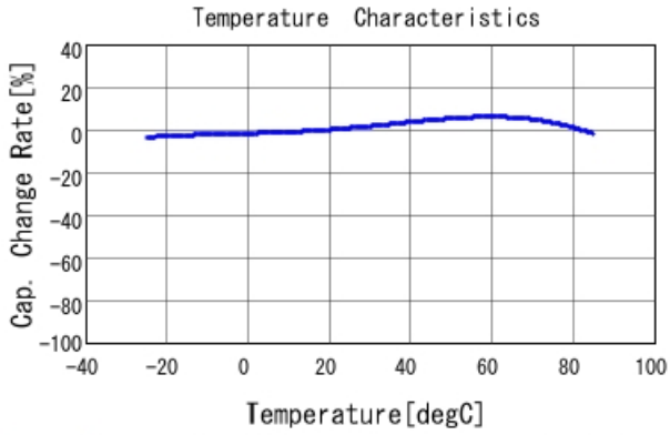
GRM32EB30J476ME16 C-Temp. capchange, DCO. 0V, ACO. 5
