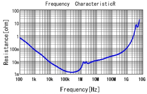
GRM32EB30J476ME16 R DCOV, 20degC
