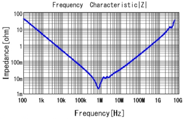
GRM32EB30J476ME16 |Z| DCOV, 20degC
