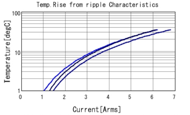
GRM32EB30J476ME16 Temp. rise — 60kHz — 300kHz
