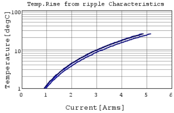
KCM55WR71E476MH01 Temp.rise — 50kHz
