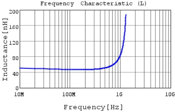
LQG18HH47NJ00 L
