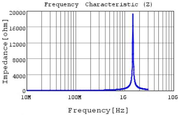
LQG18HH47NJ00 |Z|
