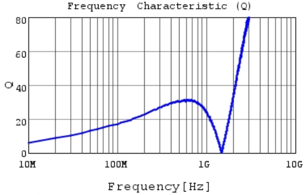
LQG18HH47NJ00 Q
