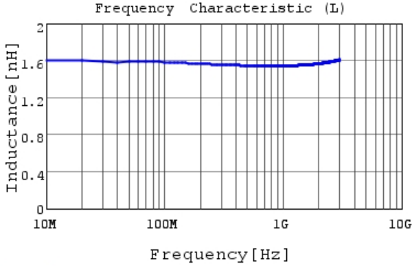
LQW15AN1N6C0Z L
