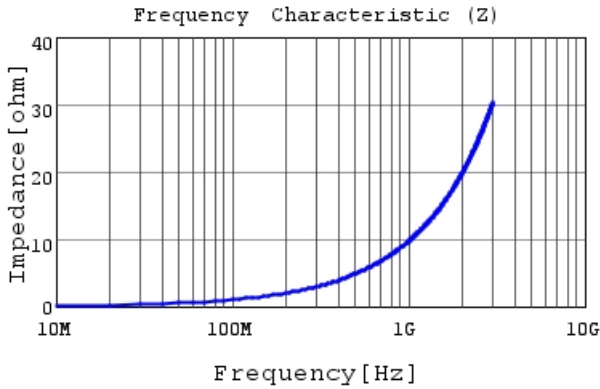
LQW15AN1N6C0Z |Z|
