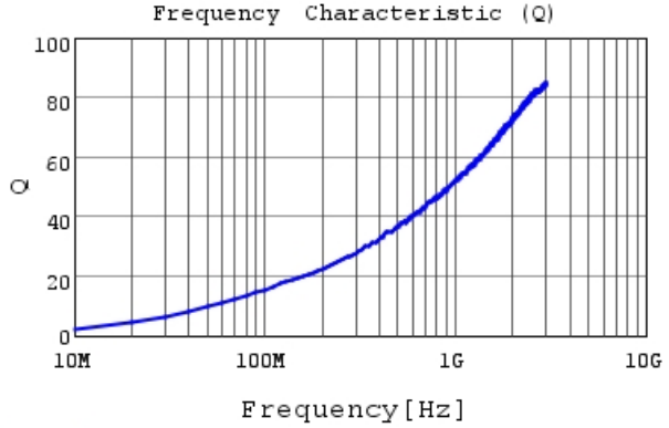
LQW15AN1N6C0Z Q
