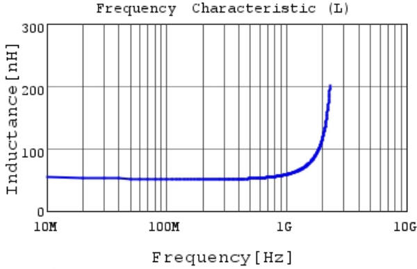
LQW18AS51NG0Z L
