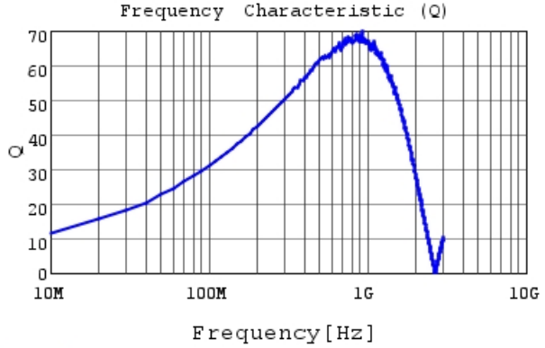
LQW18AS51NG0Z Q
