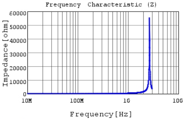
LQW18AS51NG0Z |Z|
