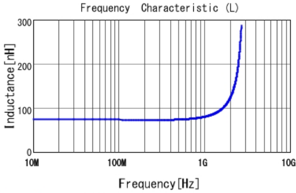
LQW15AN72NG0Z L
