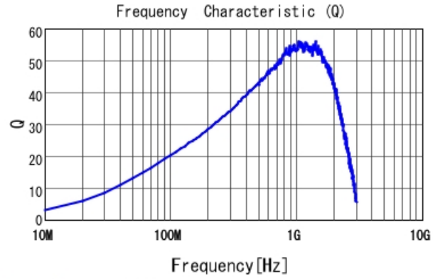
LQW15AN72NG0Z Q
