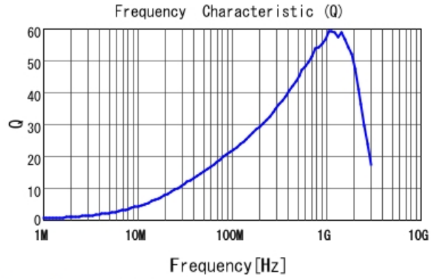
LQW15AN56NJ8Z Q
