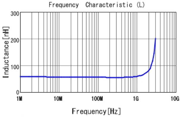
LQW15AN56NJ8Z L
