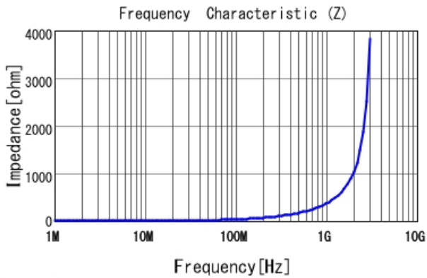
LQW15AN56NJ8Z |Z|
