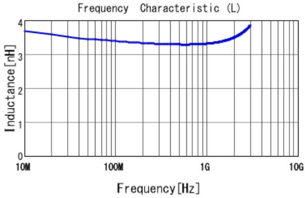
LQG15WH3N4S02 L
