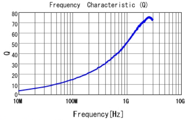
LQG15WH3N4S02 Q
