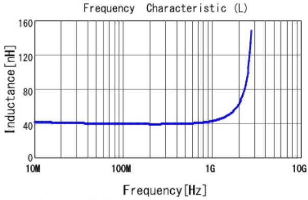
LQW18AN39NG8Z L
