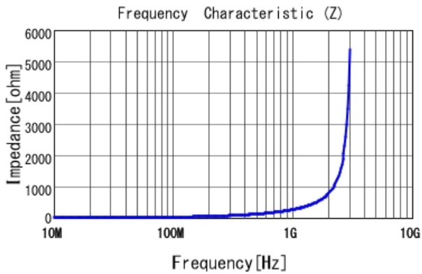
LQW18AN39NG8Z |Z|
