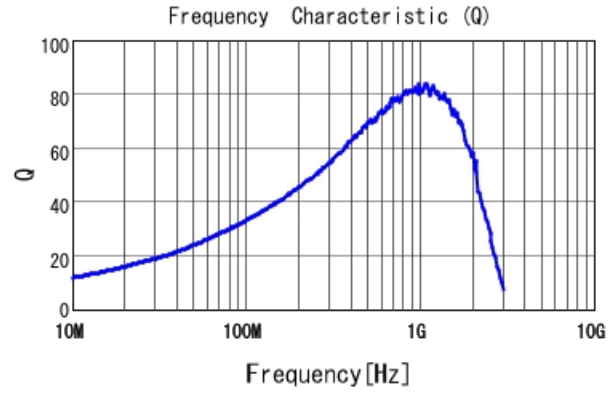
LQW18AN39NG8Z Q
