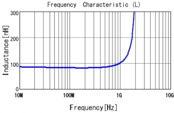
LQW18AN82NG8Z L
