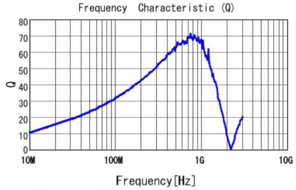
LQW18AN82NG8Z Q
