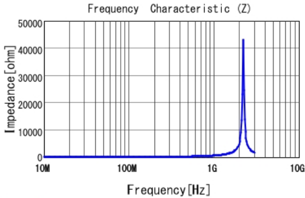
LQW18AN82NG8Z |Z|
