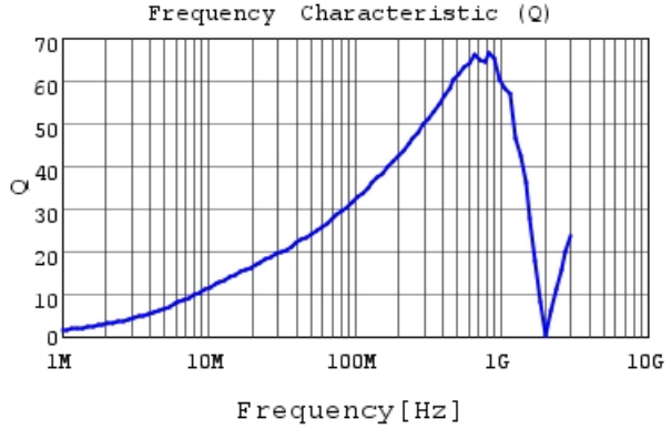
LQW18AN91NG8Z Q
