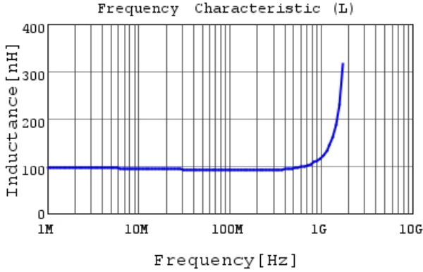
LQW18AN91NG8Z L
