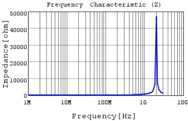
LQW18AN91NG8Z |Z|
