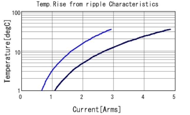
GRM21BR70J225KA01 Temp. rise — 100kHz — 500
