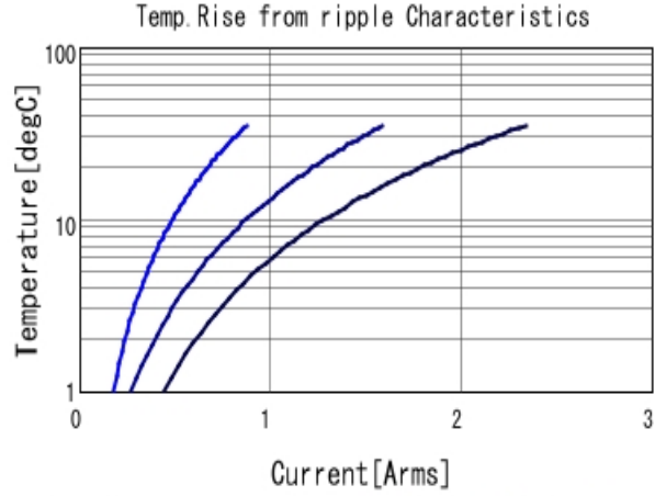
GCJ43DR72E474KXJ1 Temp. rise ■ 30kHz ■ 100kHz ■ 300kHz
