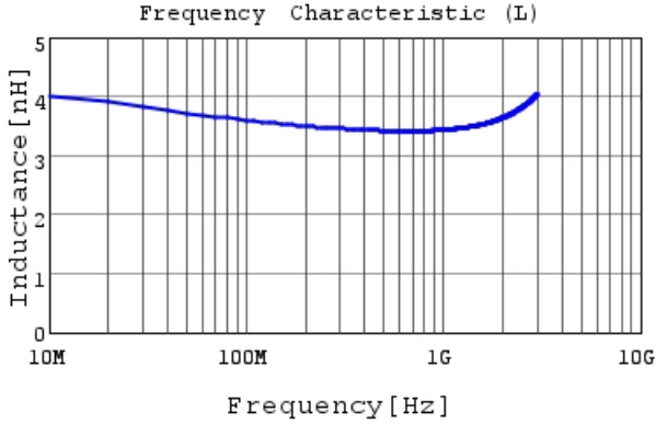
LQG15HH3N6C02 L
