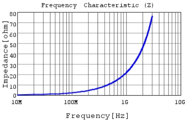
LQG15HH3N6C02 |Z|
