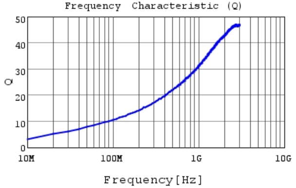
LQG15HH3N6C02 Q
