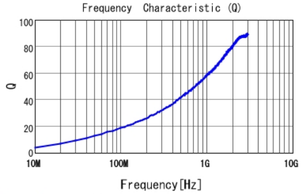
LQW15AN3N0B00 Q
