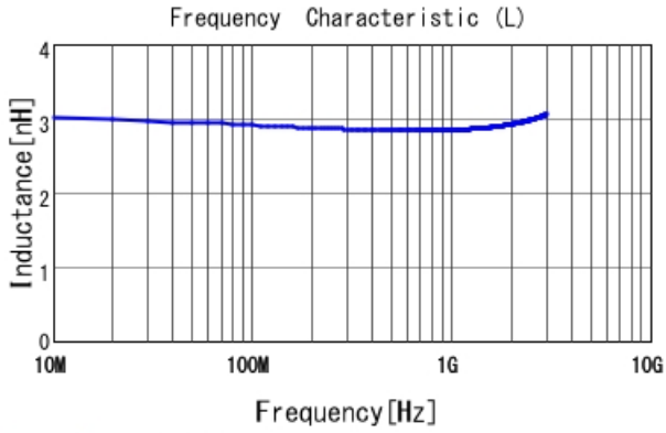
LQW15AN3N0B00 L
