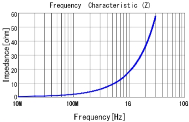
LQW15AN3N0B00 |Z|
