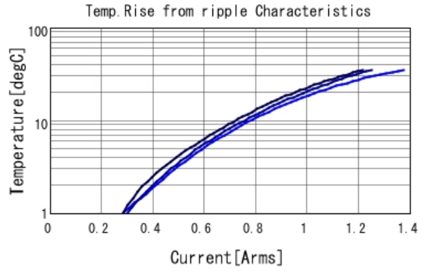
GQM2195C2E150JB12 Temp. rise — 500MHz — 700I
