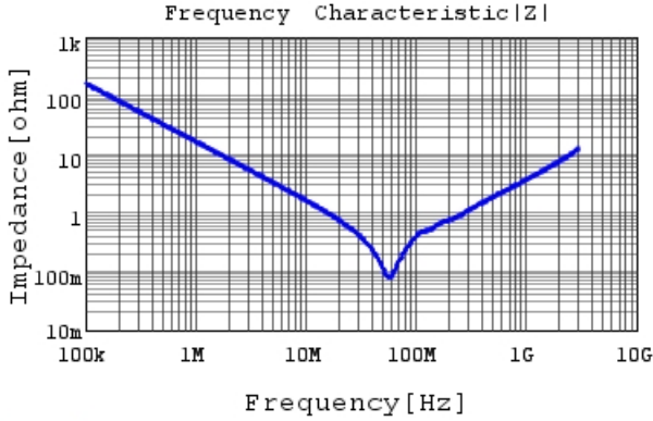
GCJ31CR73A103KXJ3 |Z| DC0V, 25degC
