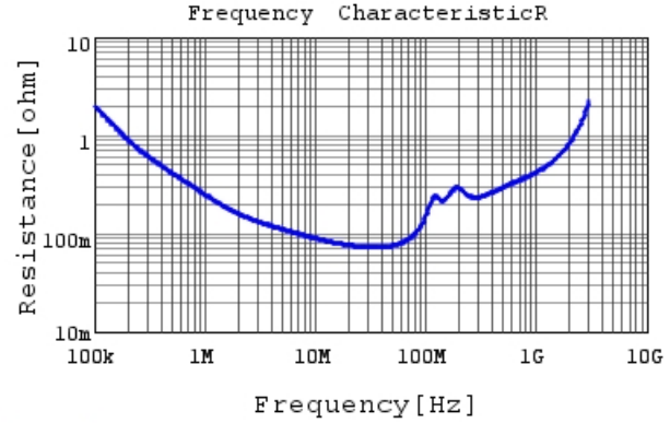
GCJ31CR73A103KXJ3 R DC0V, 25degC
