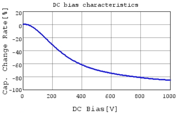
GCJ31CR73A103KXJ3 C-DC bias capchange, 25.0c
