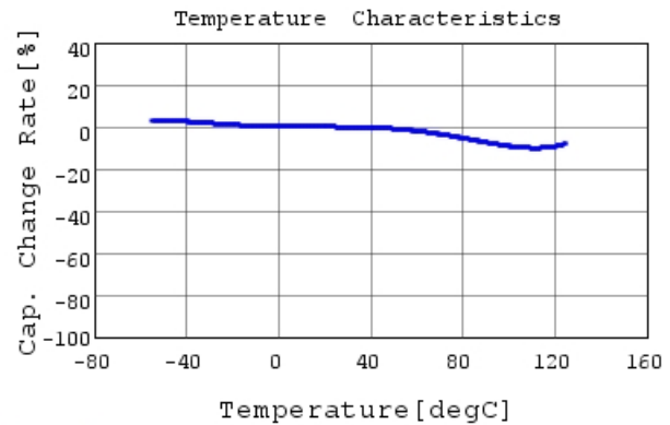
GCJ31CR73A103KXJ3 C-Temp. capchange, DC0V, 1
