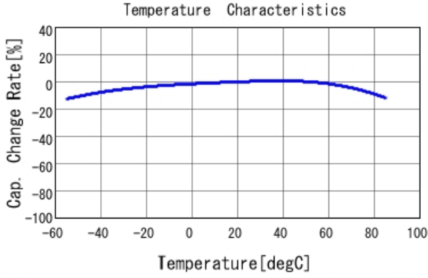
■ GRM21BR60G476ME01 C-Temp. capchange, DCO. 0V, ACO. 1Vrm
