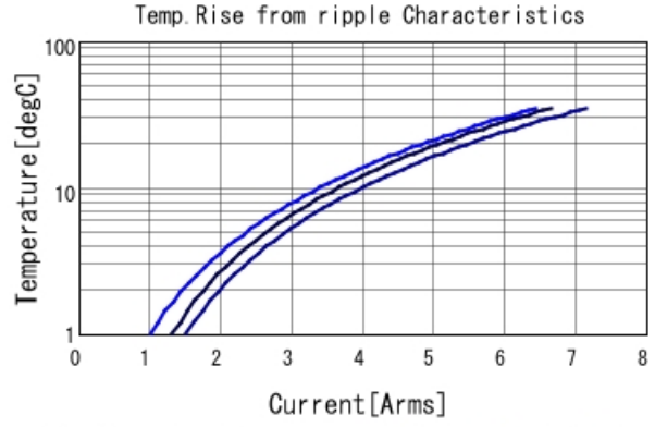
GRM21BR60G476ME01 Temp. rise ■ 60kHz ■ 300kHz ■ 600kHz
