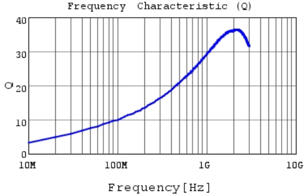
LQG15HZ6N2S02 Q
