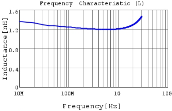
LQG15HZ1N3C02 L
