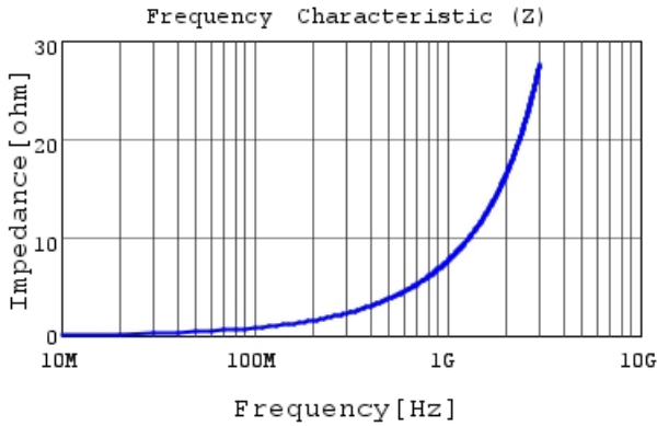
LQG15HZ1N3C02 |Z|
