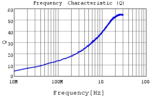
LQG15HZ1N3C02 Q
