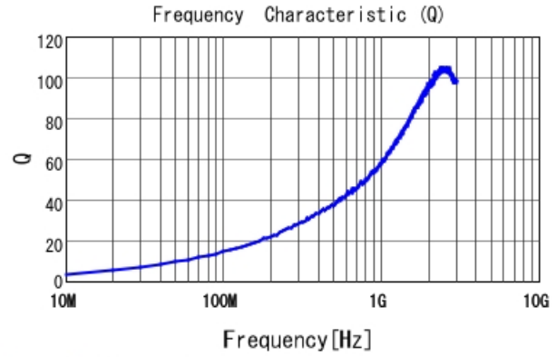
LQG15WH1N9S02 Q
