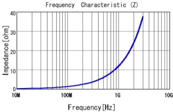
LQG15WH1N9S02 |Z|
