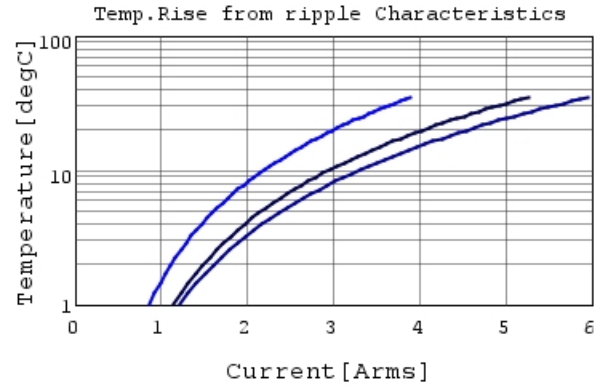
GRT32DC81H335KE01 Temp.rise — 100kHz —
