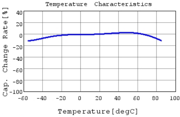
■ NFM15PC915R0E3 C-Temp. capchange, DCOV, ACO.
